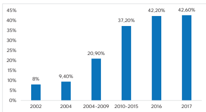
Gráfica VIII-3. Tratamiento de aguas residuales
